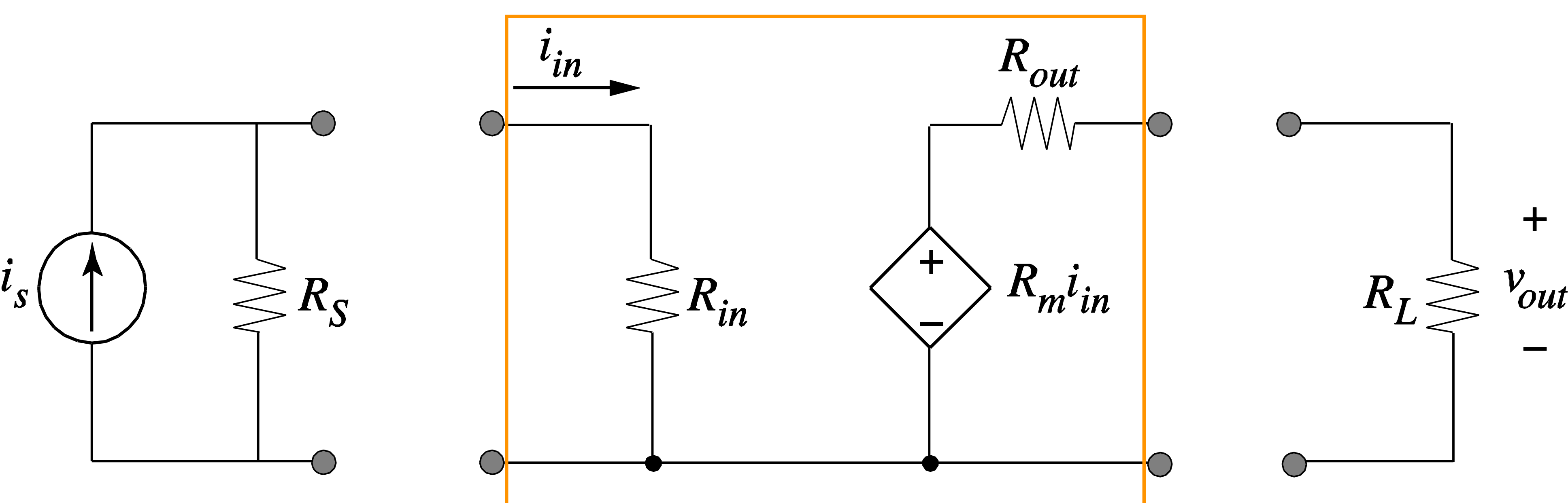
(d) Transresistance Amplifier Model
